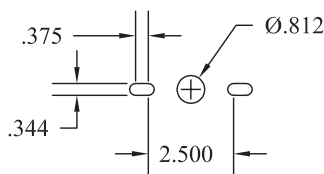
YOKE DRILLING PATTERN GABARIT DE PERÇAGE POUR L'ÉTRIER DE MONTAGE
