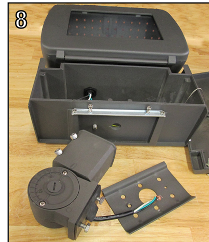
Préparer le kit d'assemblage (corps du luminaire, plaque de fixation et support de poteau).
