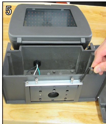
Desserrer les vis de la plaque de fixation en utilisant une clé Allen.
