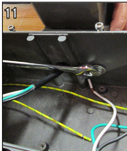
Visser le boulon qui attache le luminaire avec la plaque de fixation et le support de poteau.
