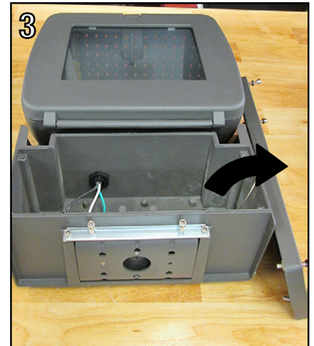
Enlever le couvercle du ballast.
