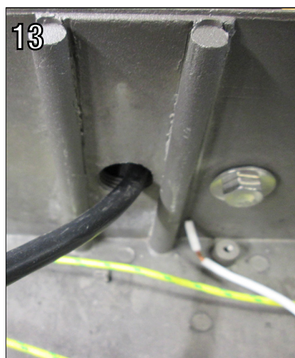
Calfeutrer l'orifice du filage électrique, pour garder l'étanchéité du luminaire.
