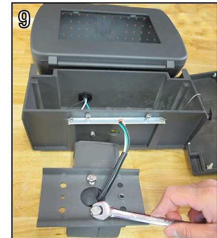
Visser la plaque de fixation sur le support de poteau.
