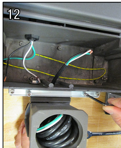
Visser les vis de la plaque de fixation en utilisant une clé Allen.
