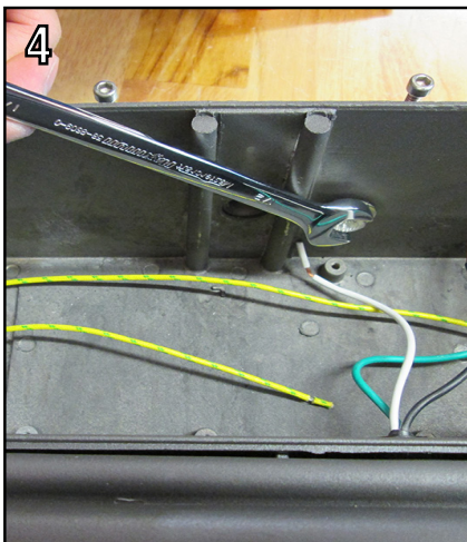
Dévisser le boulon qui retient la plaque de fixation.
